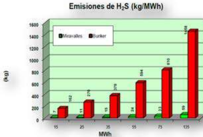
Figura 38: Emisiones de H 2 S (kg/MWh) utilizando diferentes tecnologías de generación.
