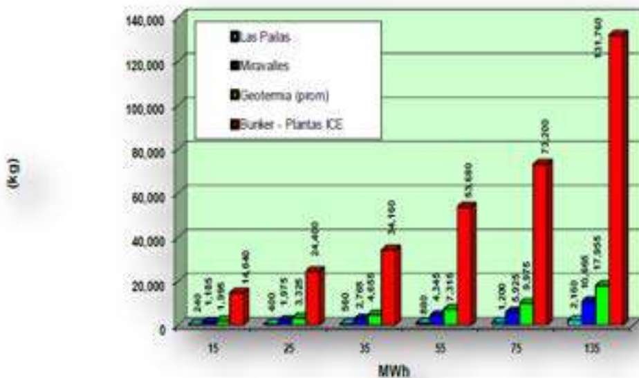
Figura 37: Emisiones de CO 2 utilizando diferentes tecnologías de generación.
